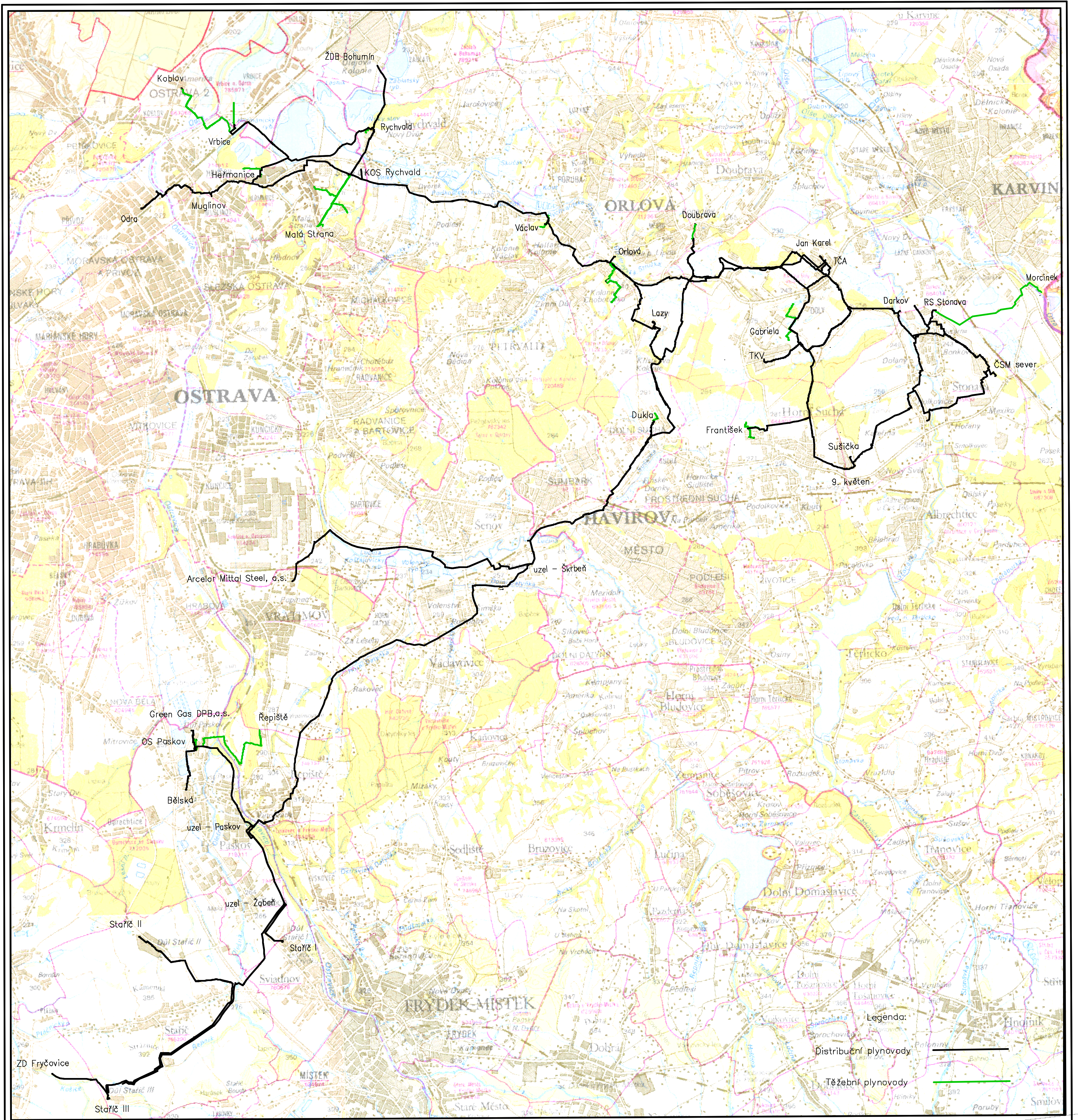
Schéma plynovodů degazačního plynu
